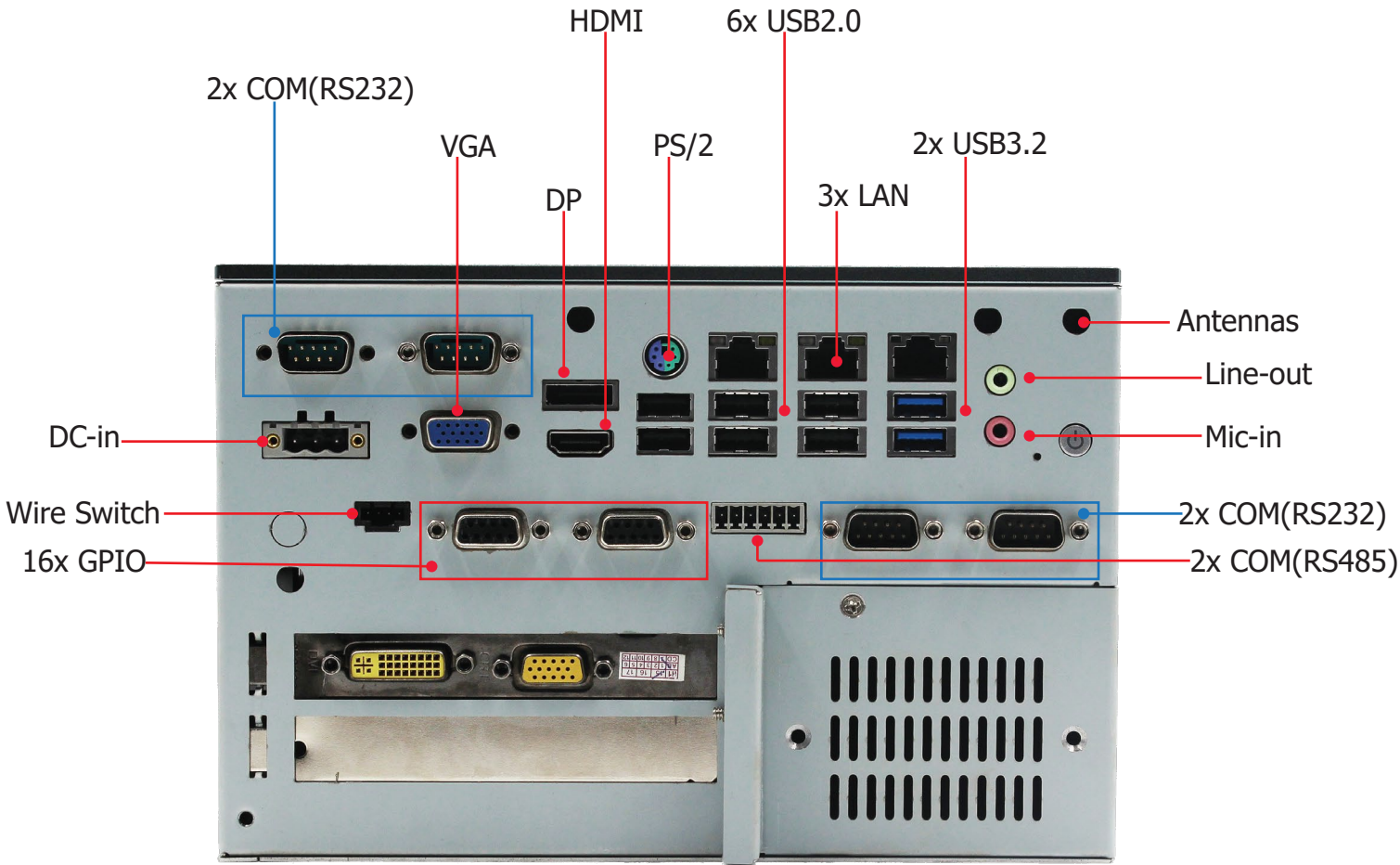
GPIO
